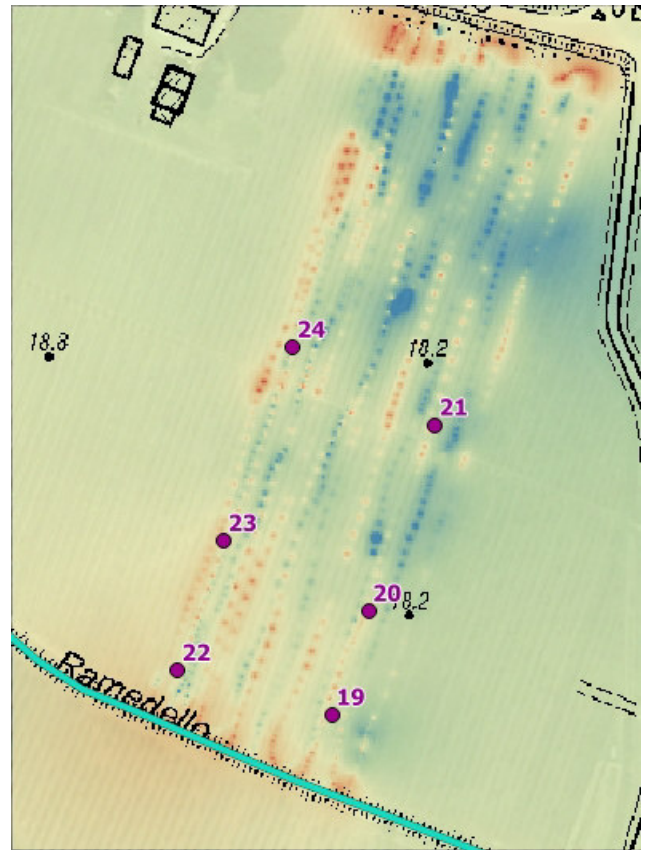
Figura 33: rappresentazioni IDW dell'andamento di conducibilità elettrica rilevata con EM38 nel sito di S. Felice s. P. nel 2018: 01/06/2018 (a sin.), 31/07/2018 (a des.), A sinistra la scala colorimetrica utilizzata (valori in milliSiemens/m).
